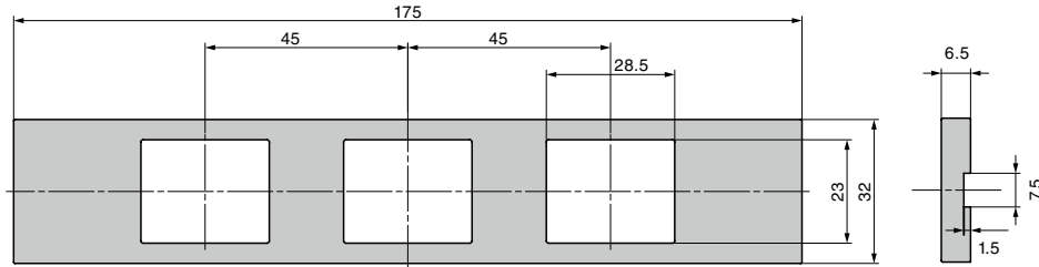
DMF3-ES (3 outlets)
