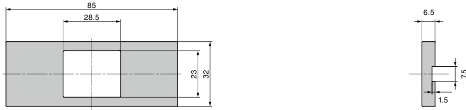
DMF1-ES (1 outlet)
