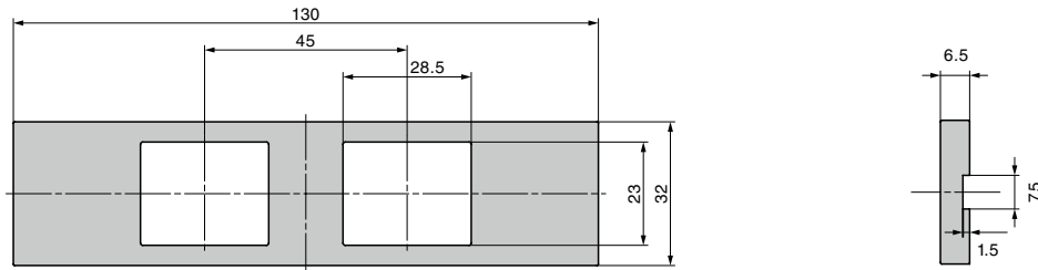
DMF2-ES (2 outlets)
