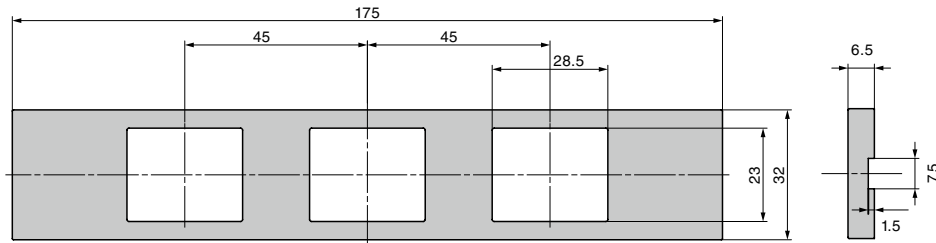
DMF3-ES (3 outlets)
