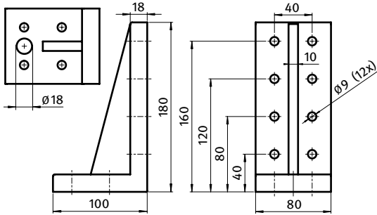
Verstiefungswinkel 80 × 180 Support bracket 80 × 180
