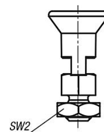
Provedení D s aretační drážkou, s protimaticí
