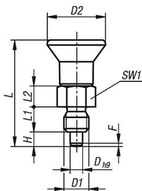
Provedení A bez aretační drážky, bez protimatice
